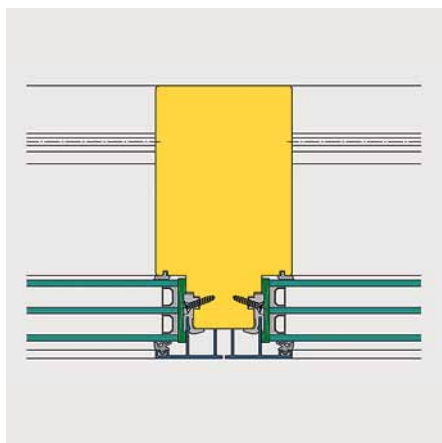
Horizontalschnitt Setzposten
