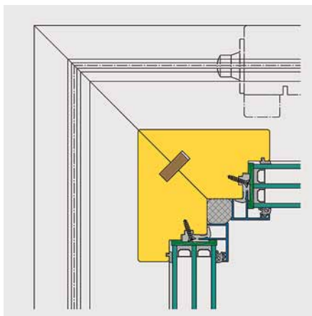
Horizontalschnitt Innenecke 90°
