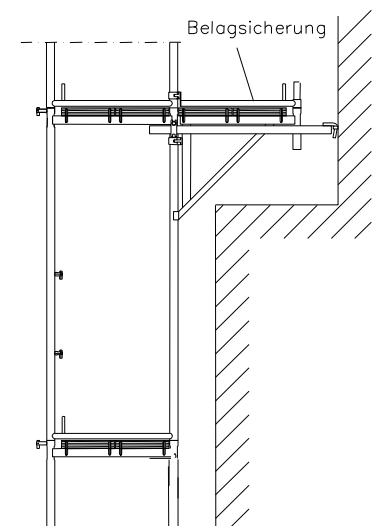
Bild 24: Konsole 64
