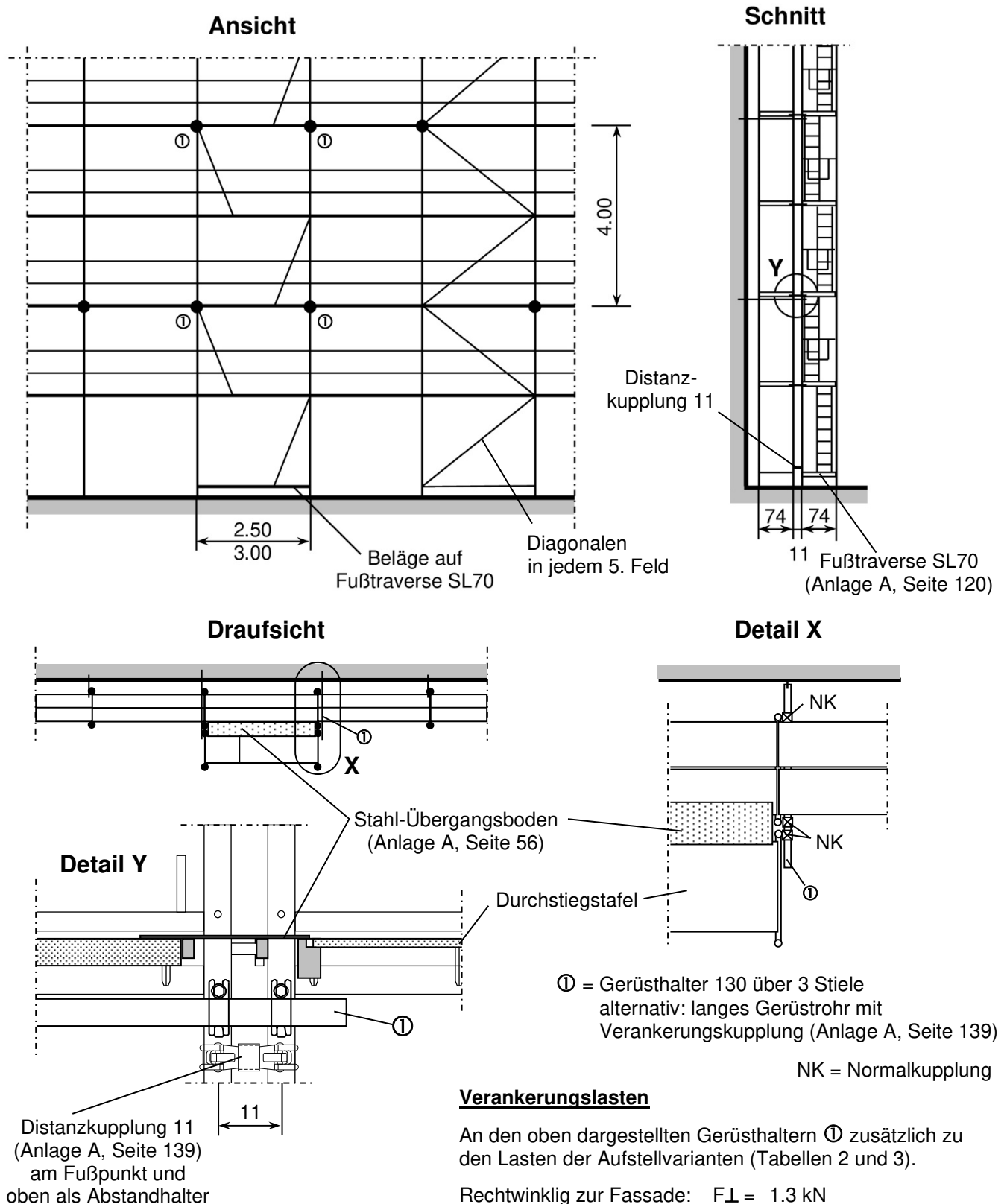
Bild 59: Leitergang
