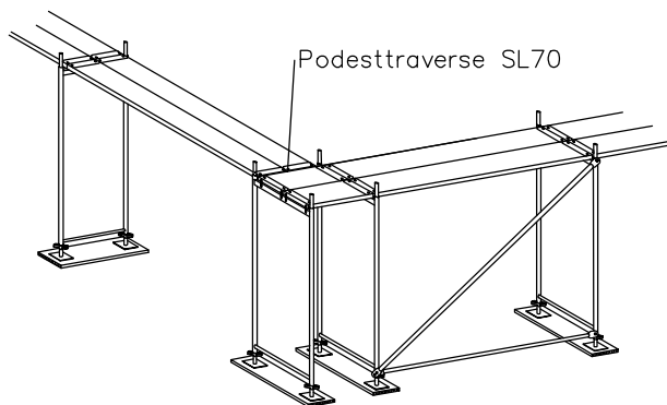
Bild 7: Eckausbildung (Variante 2)
