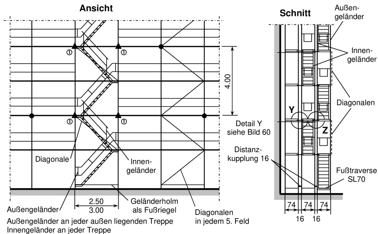
Bild 61: Gegenläufiger Treppenaufstieg
