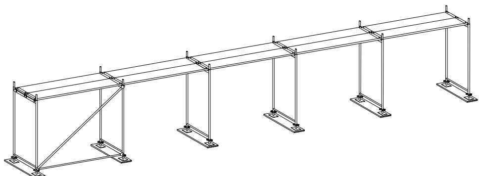
Bild 5: Einbau der Längsverstreben
