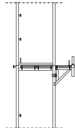
Bild 23: Konsole 32
