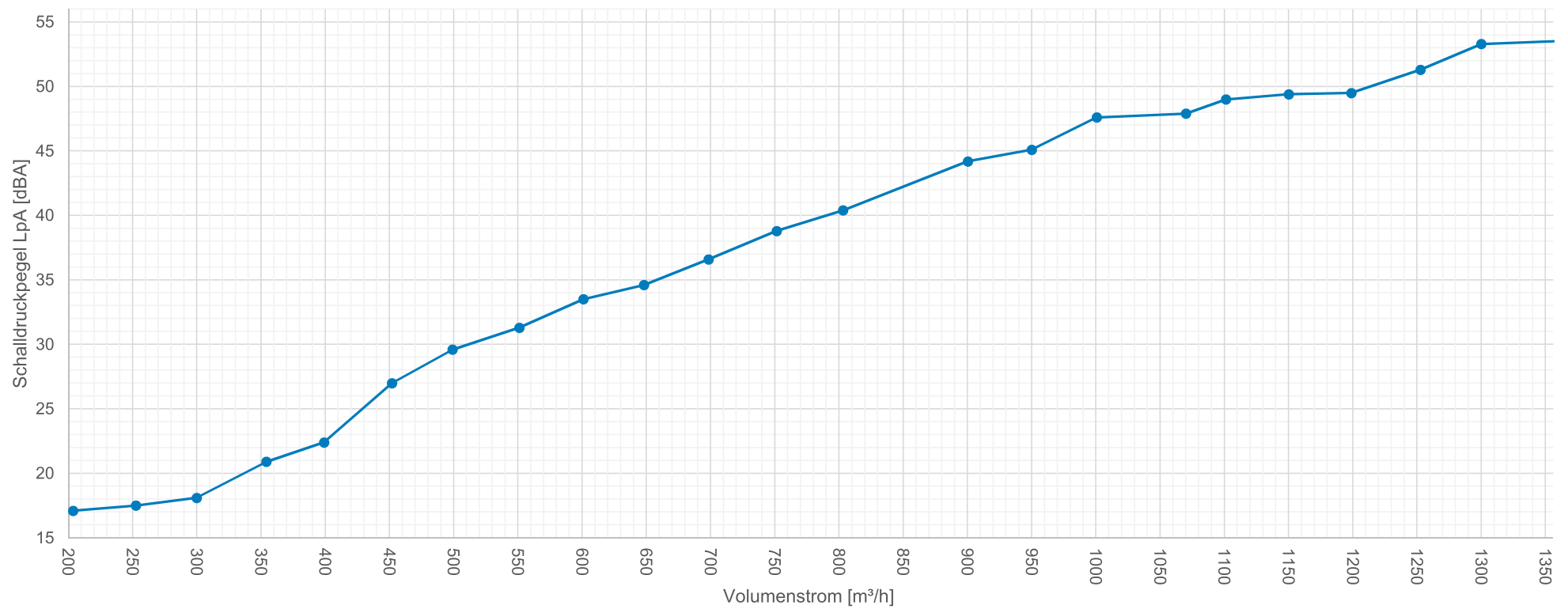
Geräuschmessung HAKA-AirClean Typ 2
