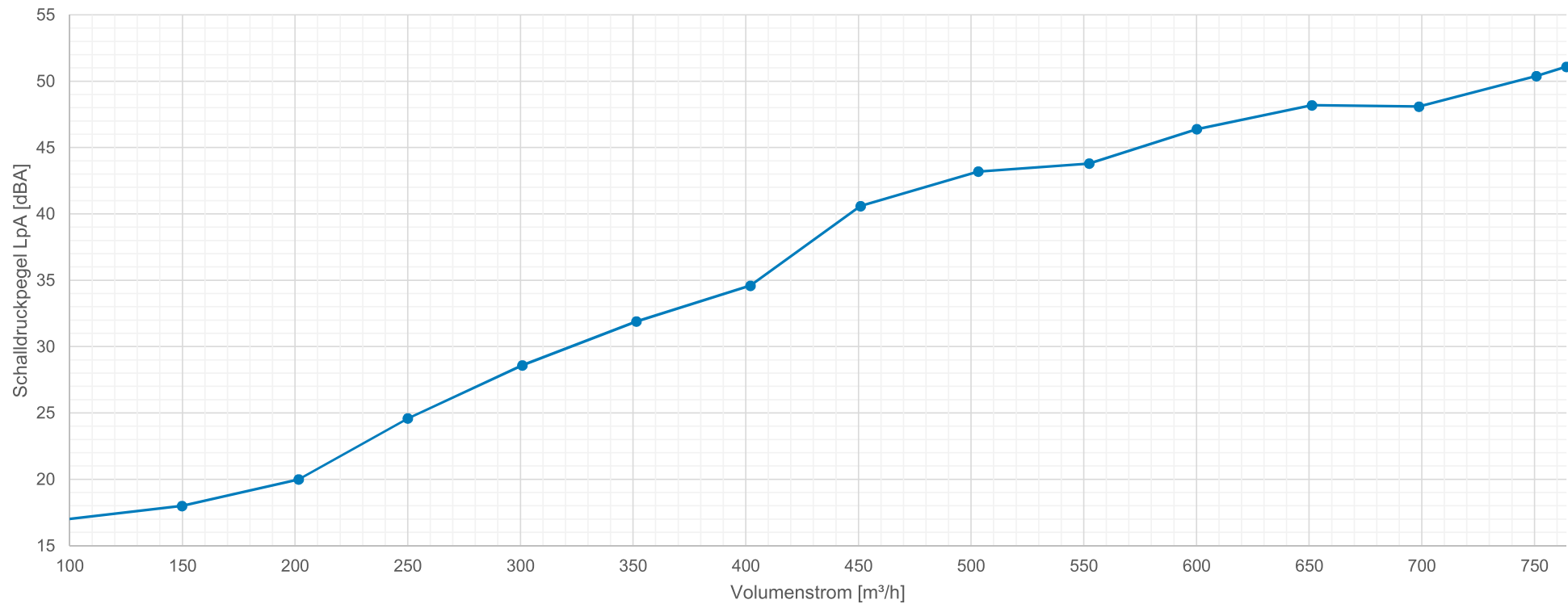
Geräuschmessung HAKA-AirClean Typ 1
