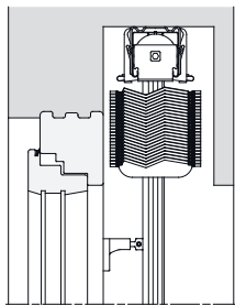
Im Schacht montiert
